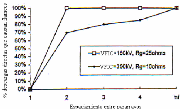
Figura 10. Espaciamiento entre pararrayos para protección contra descargas directas.
