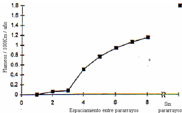
Figura 9. Espaciamiento entre pararrayos para flameos de voltajes inducidos.
