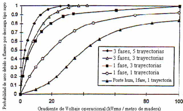
Figura 6. Probabilidad de un arco de potencia debido a un flameo por descarga tipo rayo sobre una cruceta de madera húmeda
