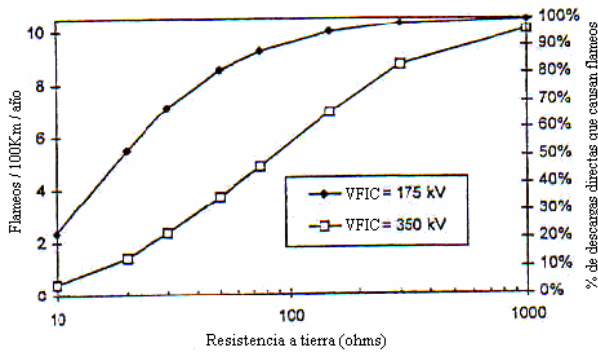
Figura 8. Efecto de la resistencia de puesta a tierra sobre el comportamiento del diseño de cable de guarda (descargas directas)
