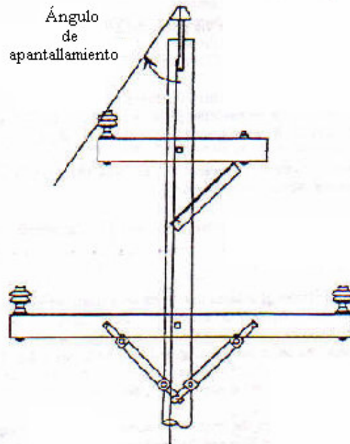
Figura 7. Ángulo de apantallamiento del cable de guarda.
